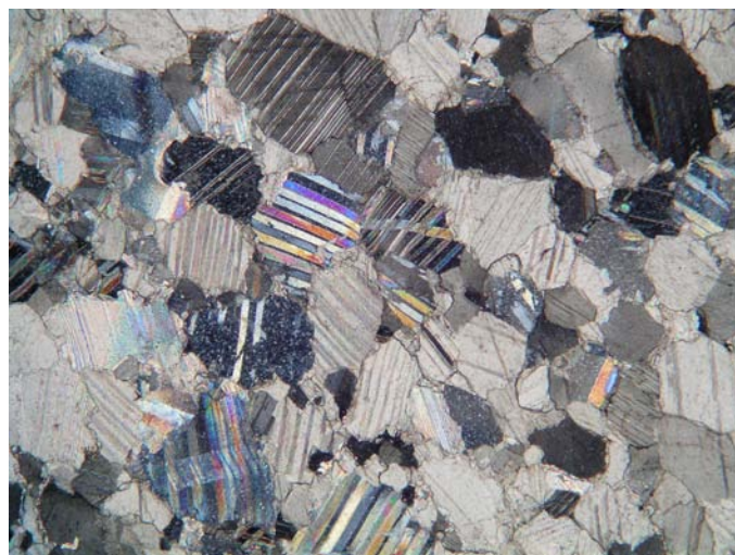
Fotografia realitzada amb microscopi de llum polaritzada plana d'una mostra de marbre del Proconnès a 60 augments (nicols creuats).
