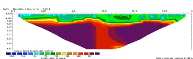
Perfil 4
