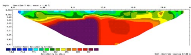
Perfil 3
