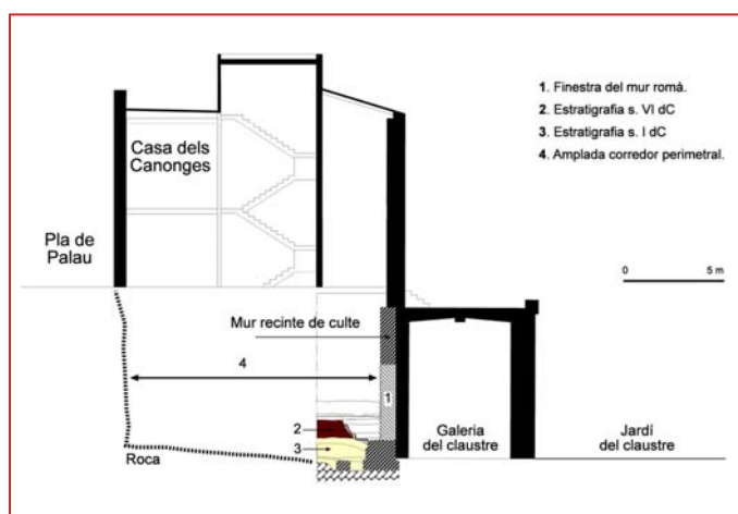
Secció dels treballs efectuats en el subsòl de la Casa dels Canonges.
