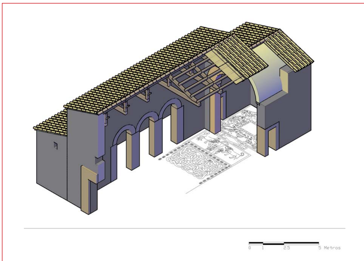
Reconstrucció de l'església de Fornàs (Menorca).
