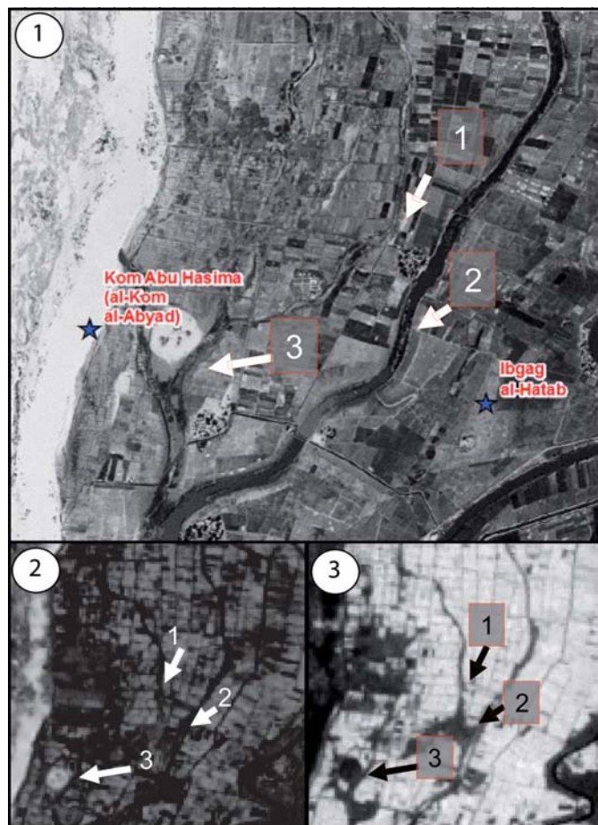
Àrea situada a 7 quilòmetres al sud d'Oxirinc. Imatge Corona, anàlisi amb índexs NDVI i traces de canals d'inundació reblerts.
