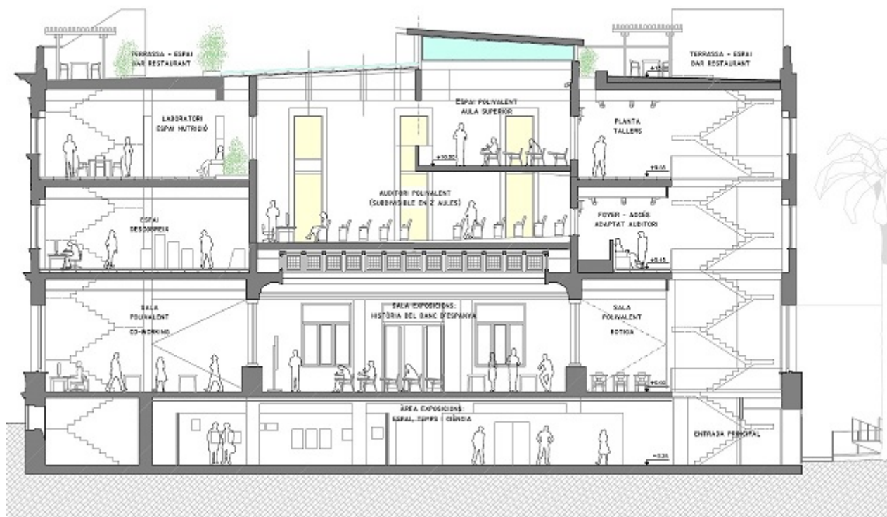
Tall longitudinal del projecte del Banc d'Espanya, amb els diferents espais (imatge: diari digital Tarragona 21)
